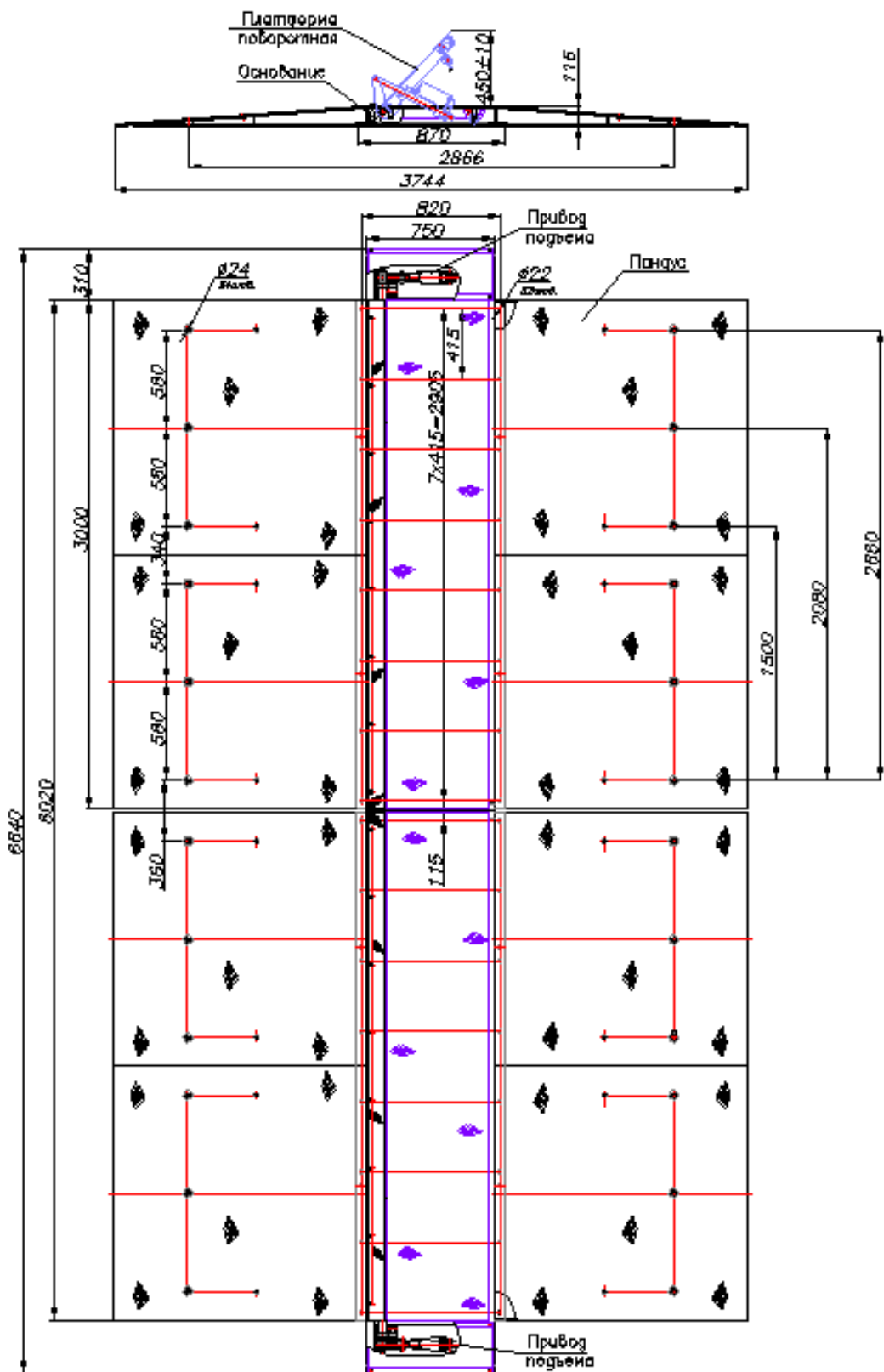
Рисунок 1. ПЗП-6000эм накладного монтажа.
