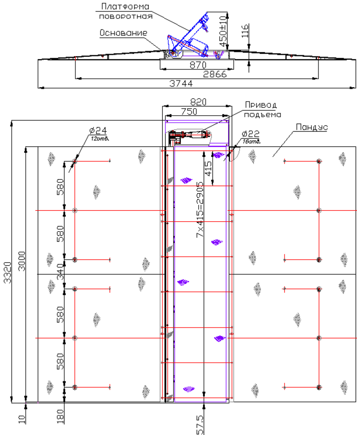
Рисунок 2. ПЗП-3000эм накладного монтажа правого исполнения.
