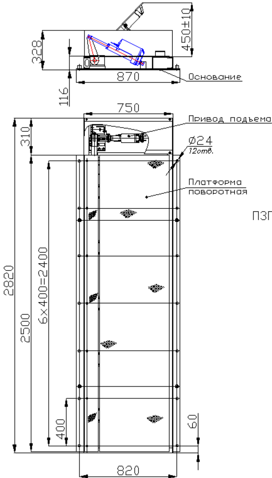
Рисунок 1. ПЗП 2500 ЭМЗ
