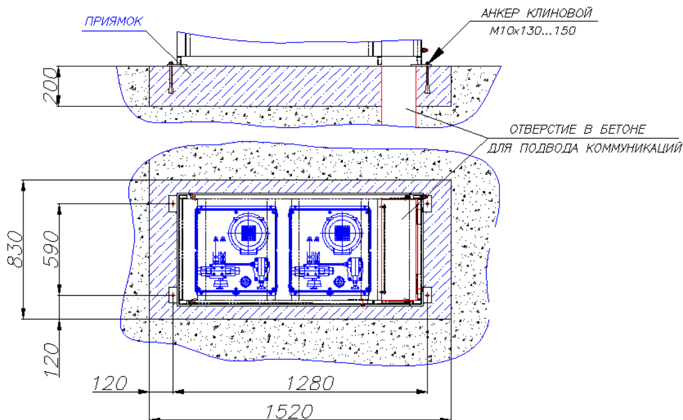
Рисунок А.1 Монтажно-установочная схема бокса
