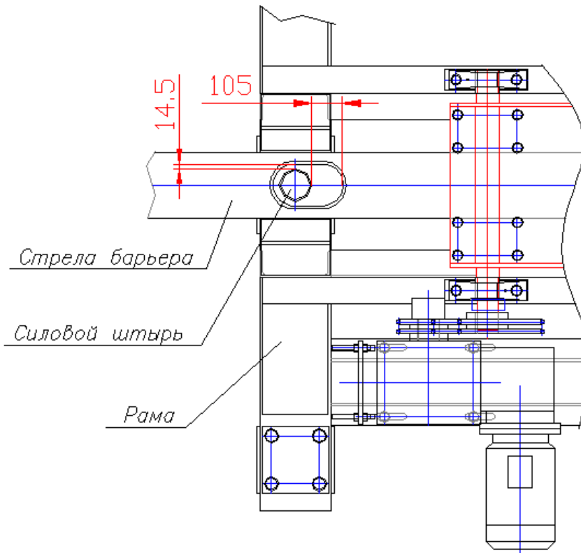
Рисунок В.4 - Зазоры между гильзой стрелы барьера и силовым штырем рамы.
