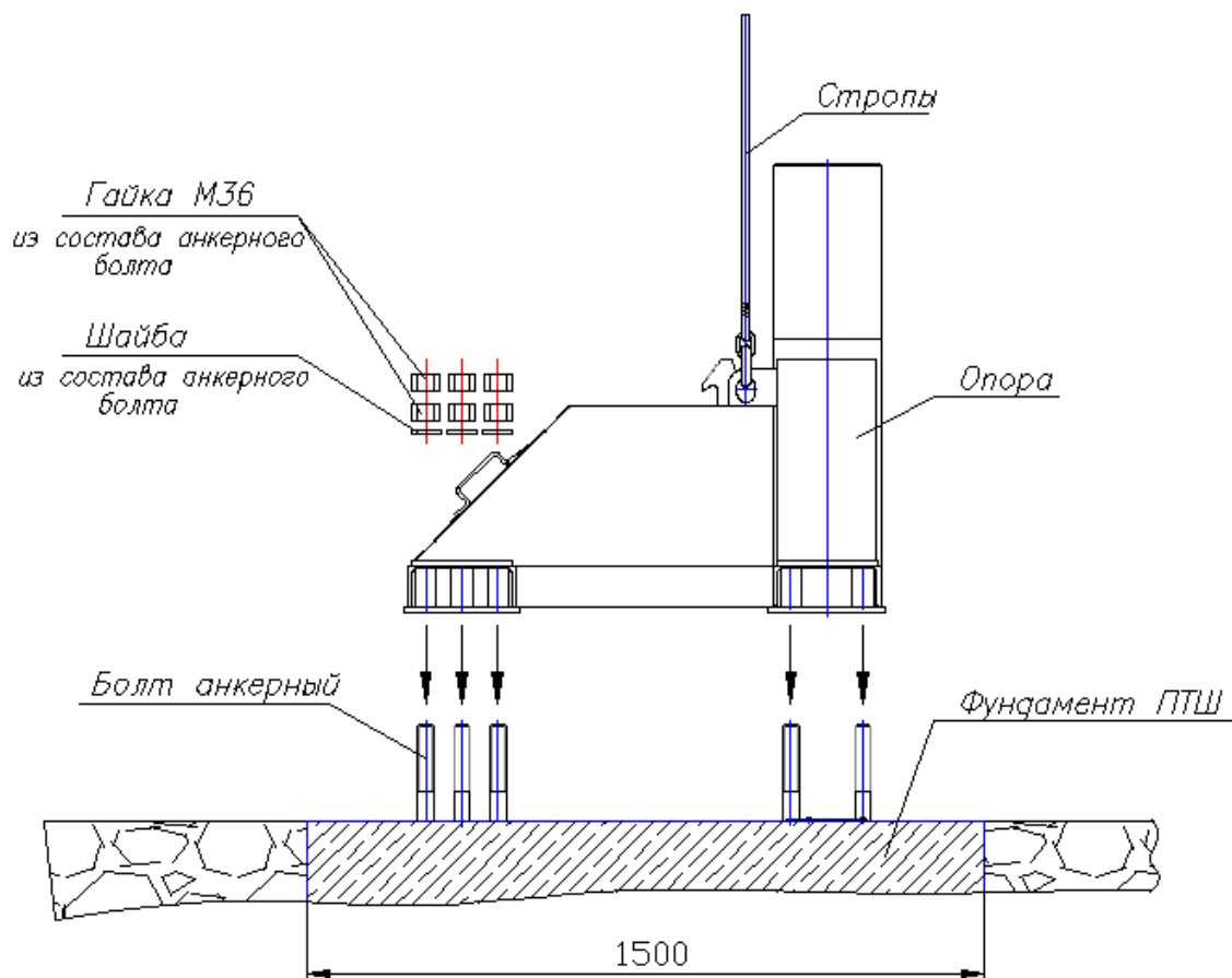
Рисунок В.1 - Установка опоры.
