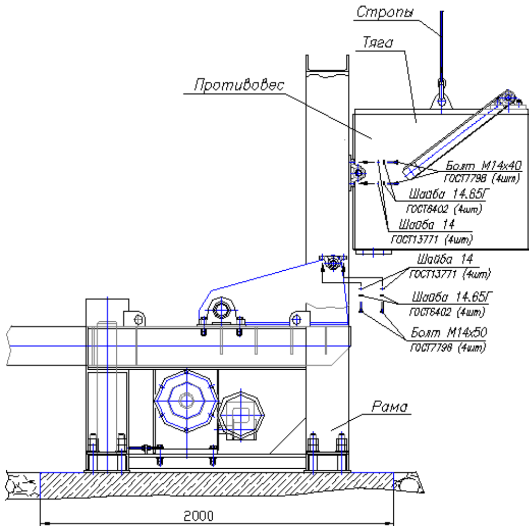
Рисунок В.5 - Установка противовеса.
