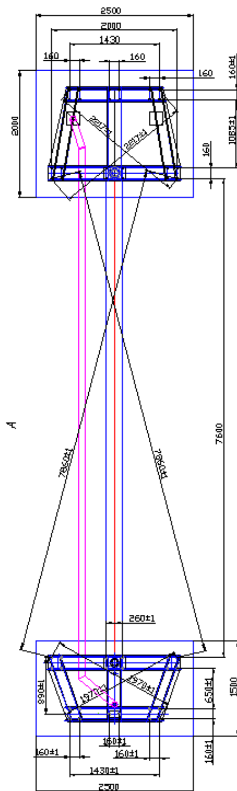
Рисунок Б.1- План фундаментных болтов ПТШ7500.
