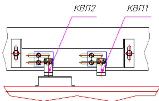
Рисунок В.6 - Установка датчиков конечных положений.
