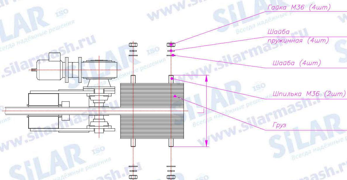
Рисунок Б.5 Противовес
