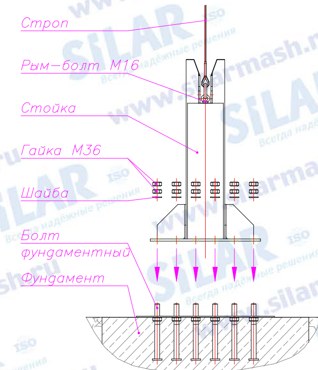
Рисунок Б.2 - Установка стойки.
